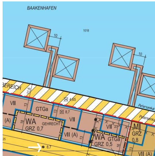
Abbildung 2 Festsetzung der Straßenhöhe bezogen auf NN im Bebauungsplan HafenCity 14 (Quelle: Freie und Hansestadt Hamburg 2015)
