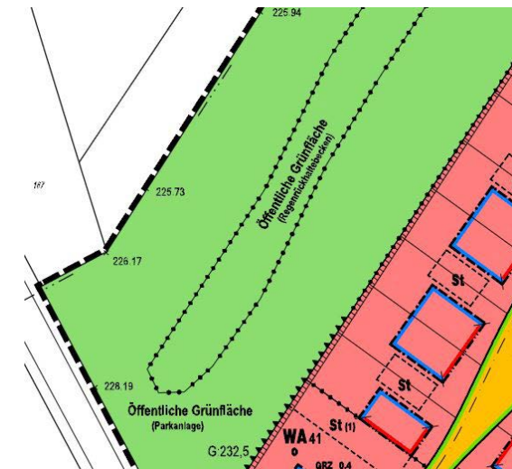
Abbildung 6 Festsetzung einer öffentlichen Grünfläche zur Regenrückhaltung im Bebauungsplan Nr. 850 der Stadt Aachen (Quelle: Stadt Aachen 2007)
